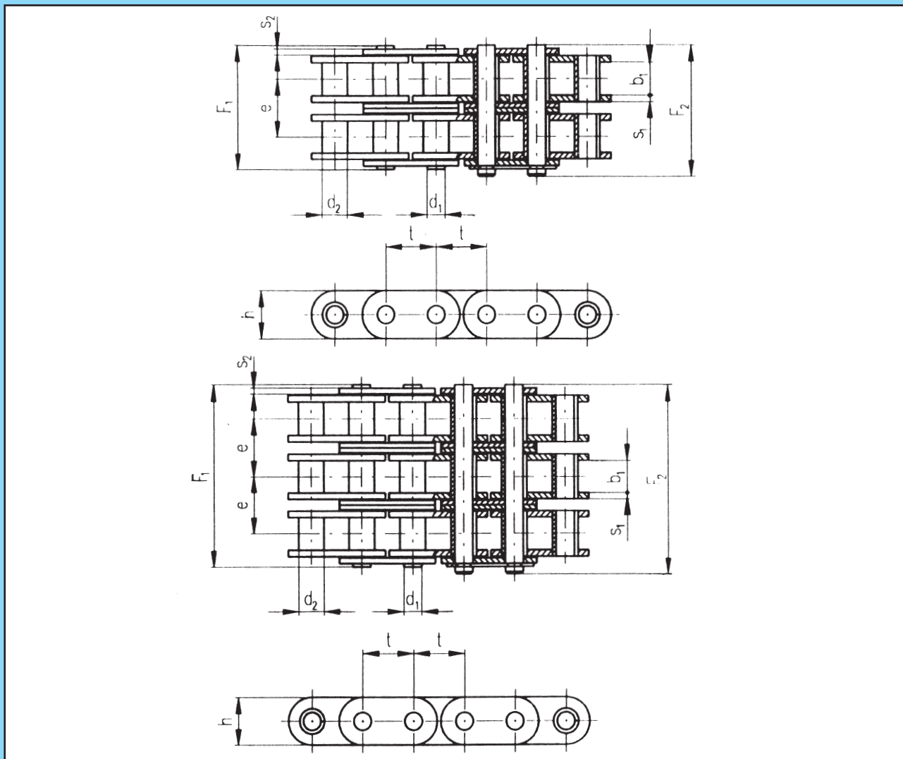
Puzdrové reťaze dvojradowé podľa ČSN 02 3321.
